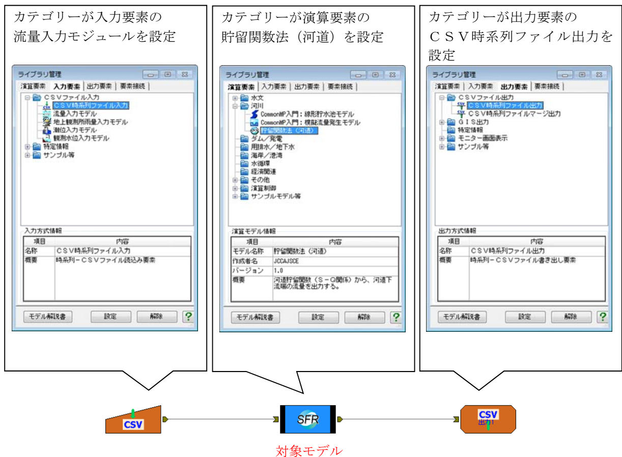
図 5 モデル接続
