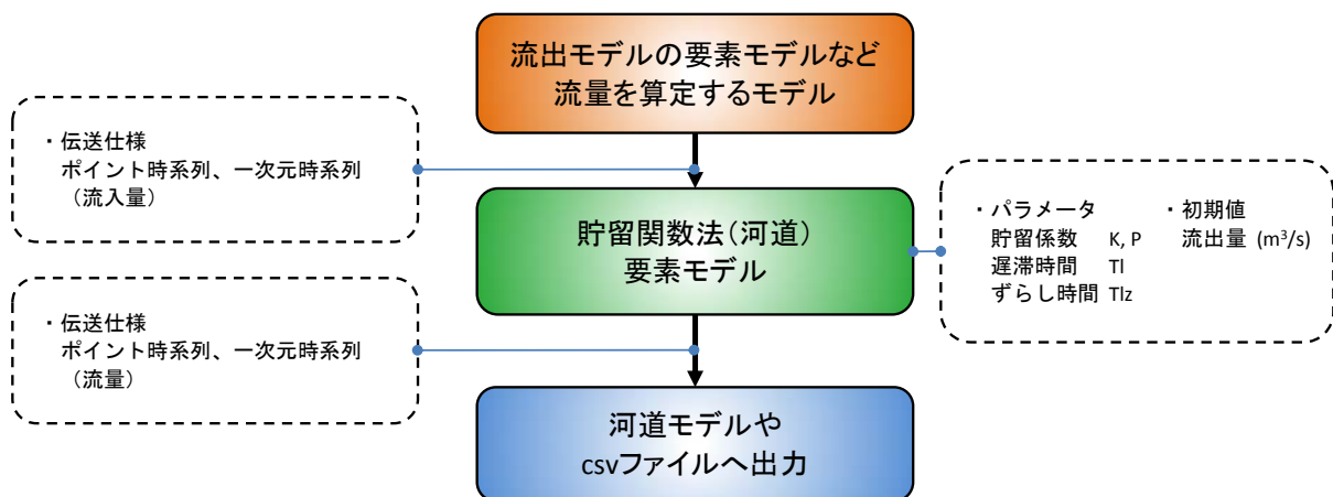
図 1 要素モデル接続概念図
